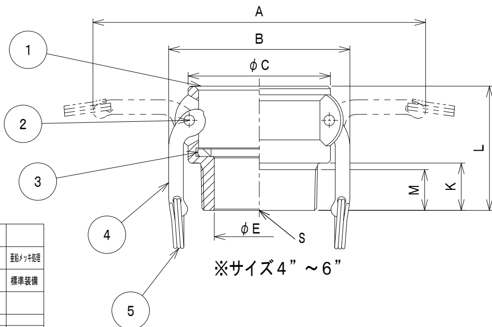
633-BB AL サイズ別寸法表 (単位: mm)
